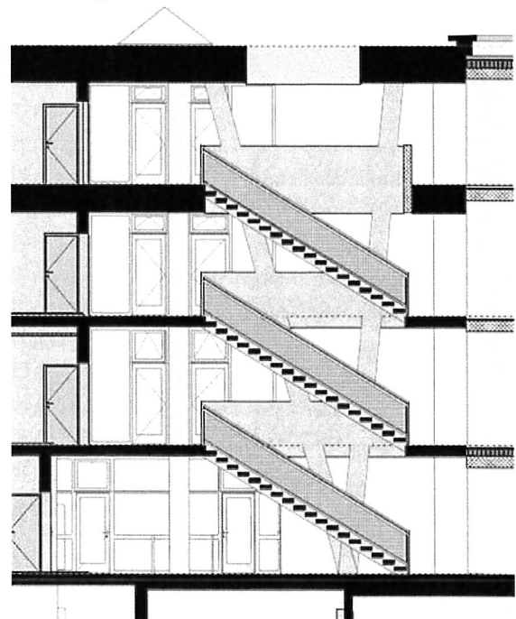
Querschnitt der neuen Haupttreppe im Eingangsbereich
